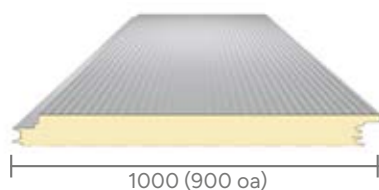
CP Superior Line Brucha ALPHA-C FX 160 mm EI60/EI60
