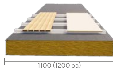
CP Superior Line Ruukki BETA CARRIER MW FX 60-300 mm Uniek FX brandwerend getest carriersysteem Mogelijk tot EI240
